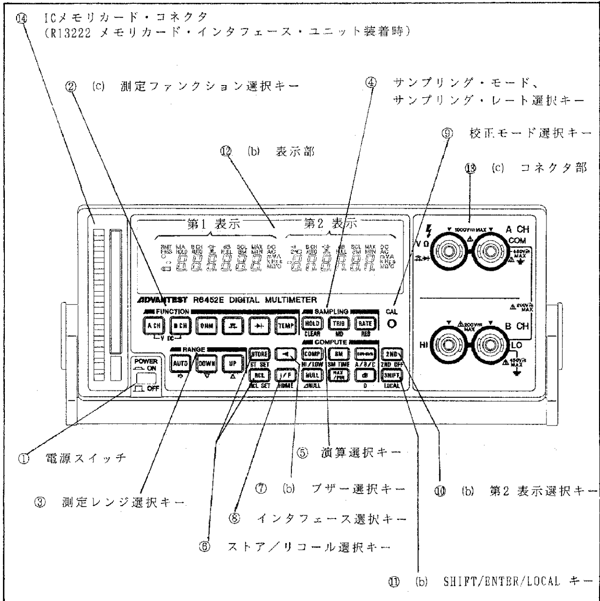
図 3 - 3 R6452E 正面パネルの説明
