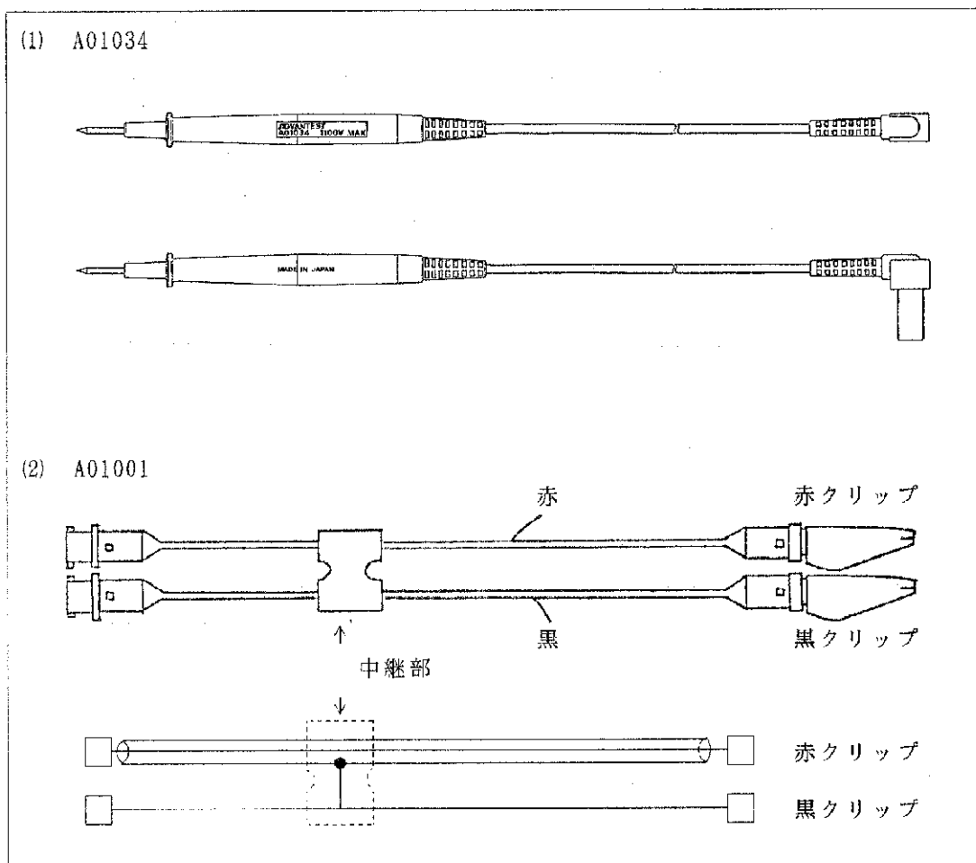
図 2 - 6 入 力 ケ ー ブ ル の 構 造
