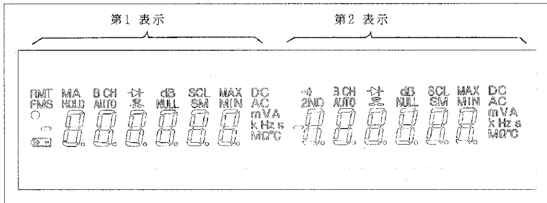
図 5 - 3 正面パネルの表示部 (R6452AとR6452Eのみ)
