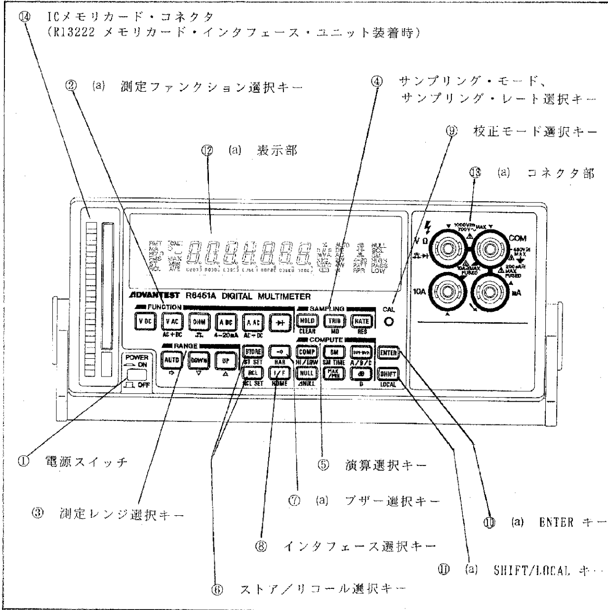
図 3 - 1 R6451A 正面パネルの説明
