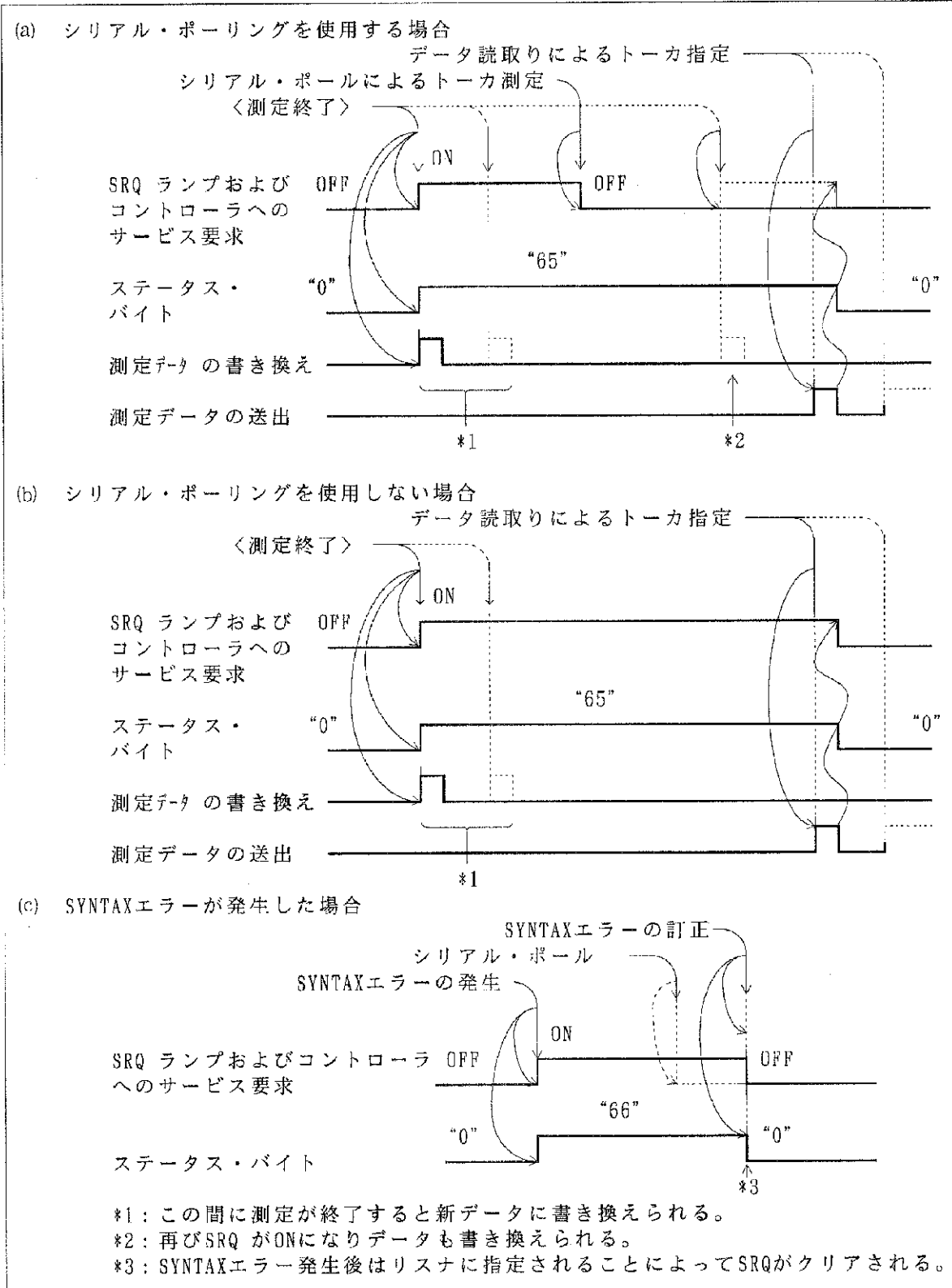
図 7 - 4 サービス要求時の動作タイミング 7 - 56
