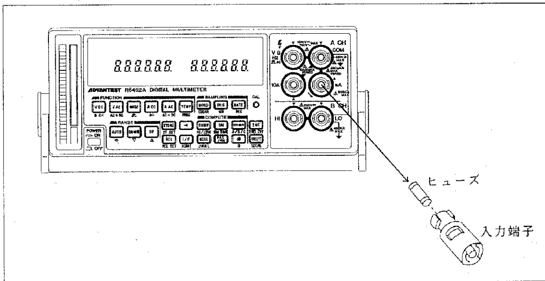
図 2 - 4 mA入力端子保護用ヒューズ
