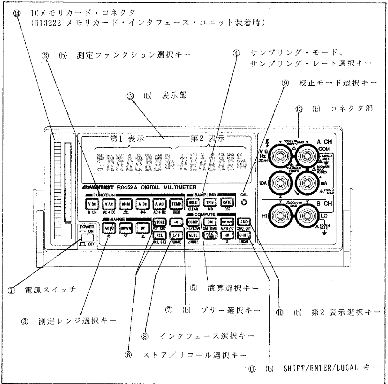
図 3 - 2 R6452A 正面パネルの説明
