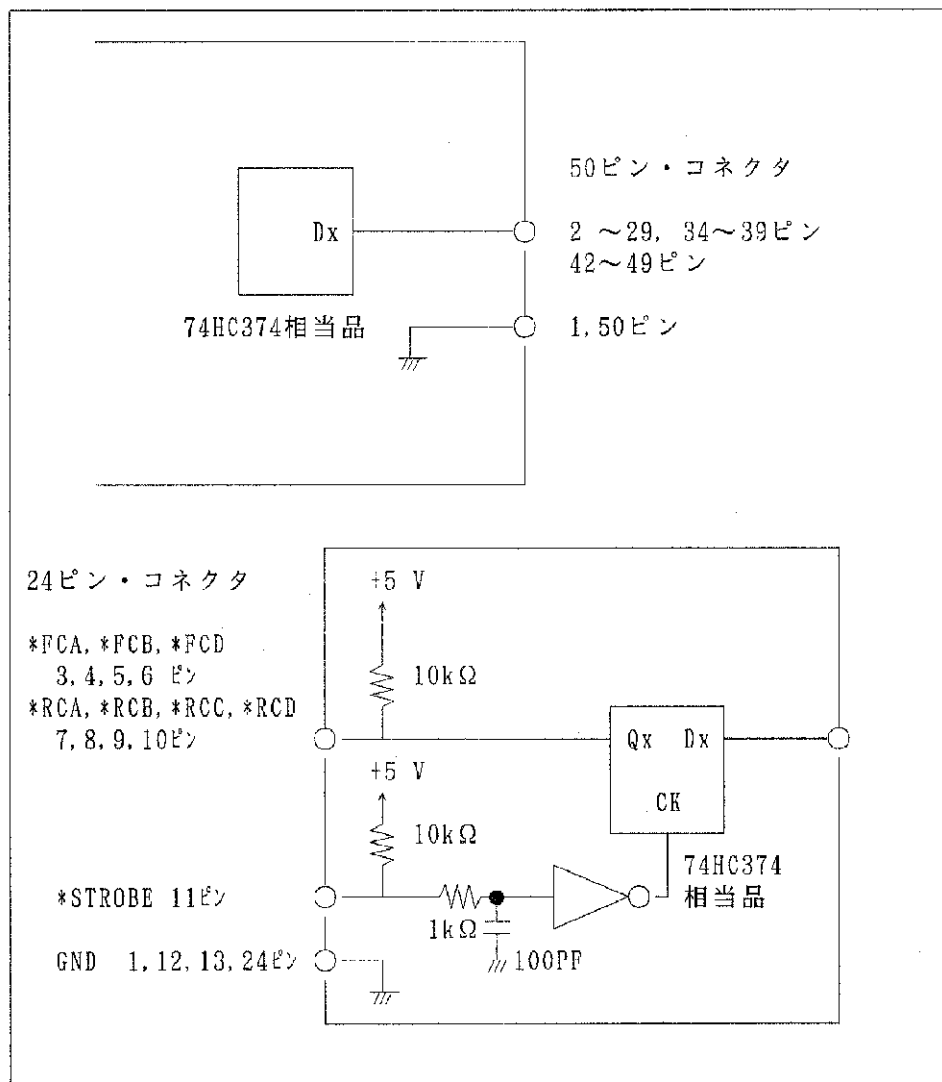
図 7 - 2 BCD 出力ユニットの出力回路、入力回路
