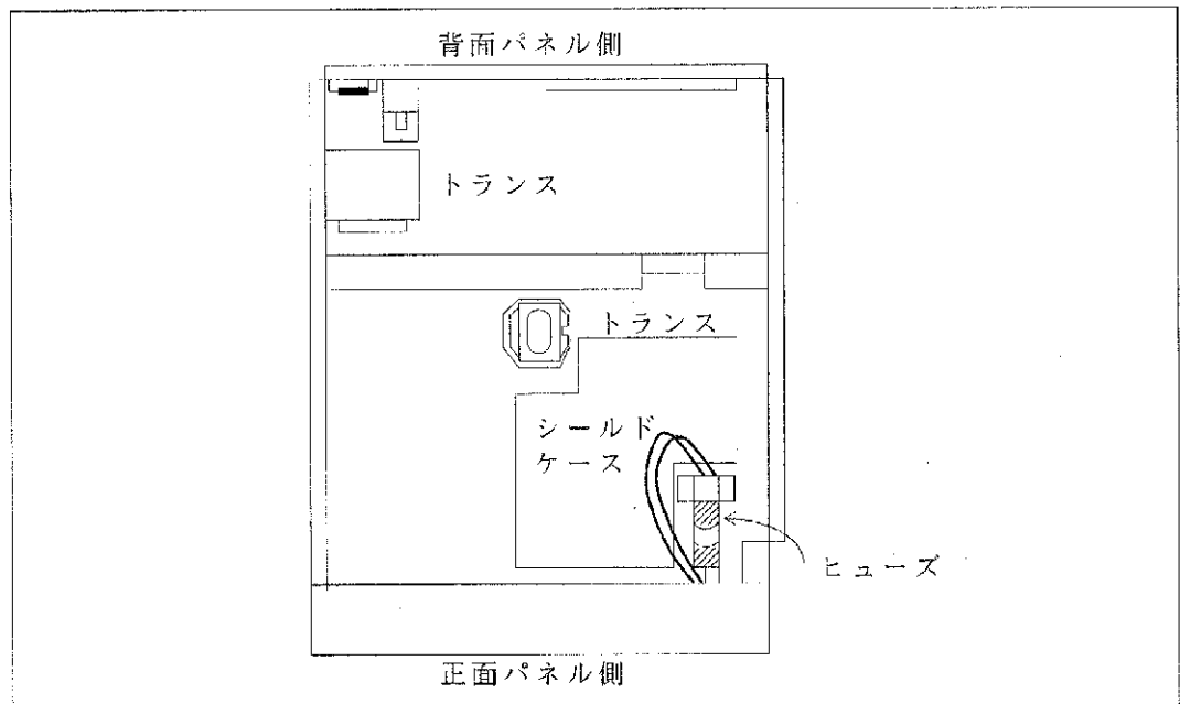
図 2 - 5 10A 入力端子保護用ヒューズ
