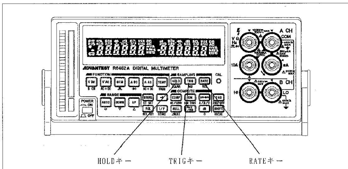
図 5 - 2 サンプリング条件の設定
